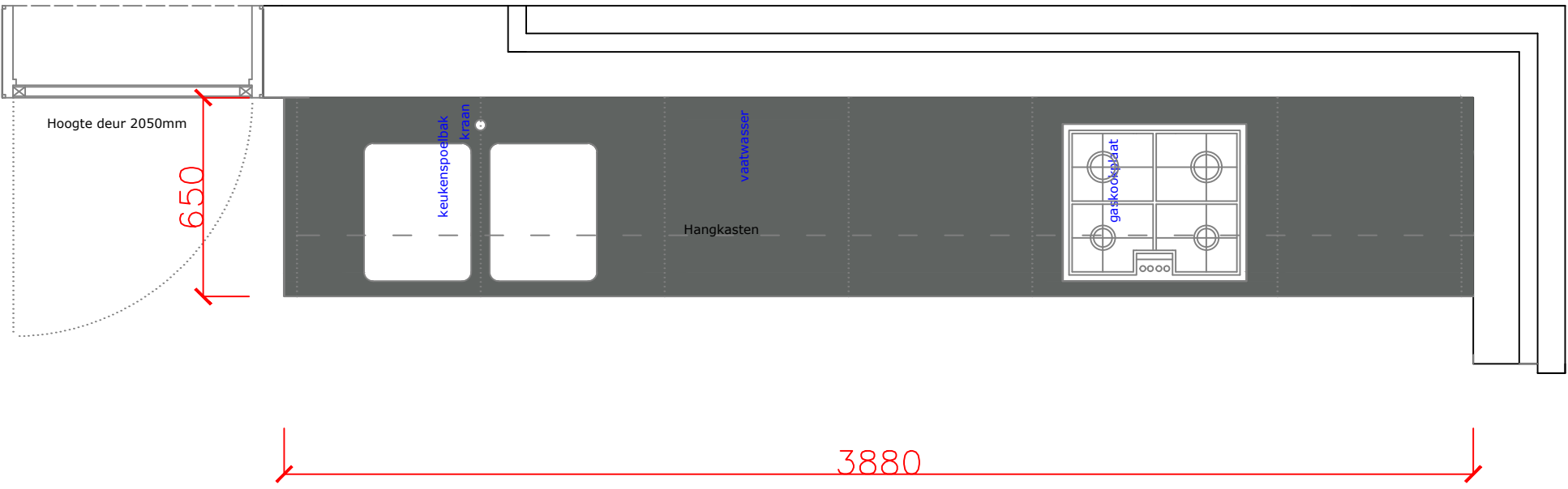
Grondplan
