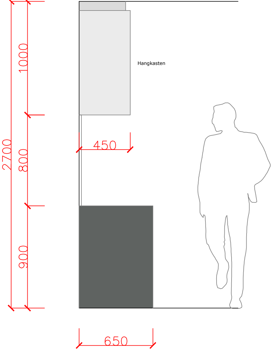
Zijaanzicht
