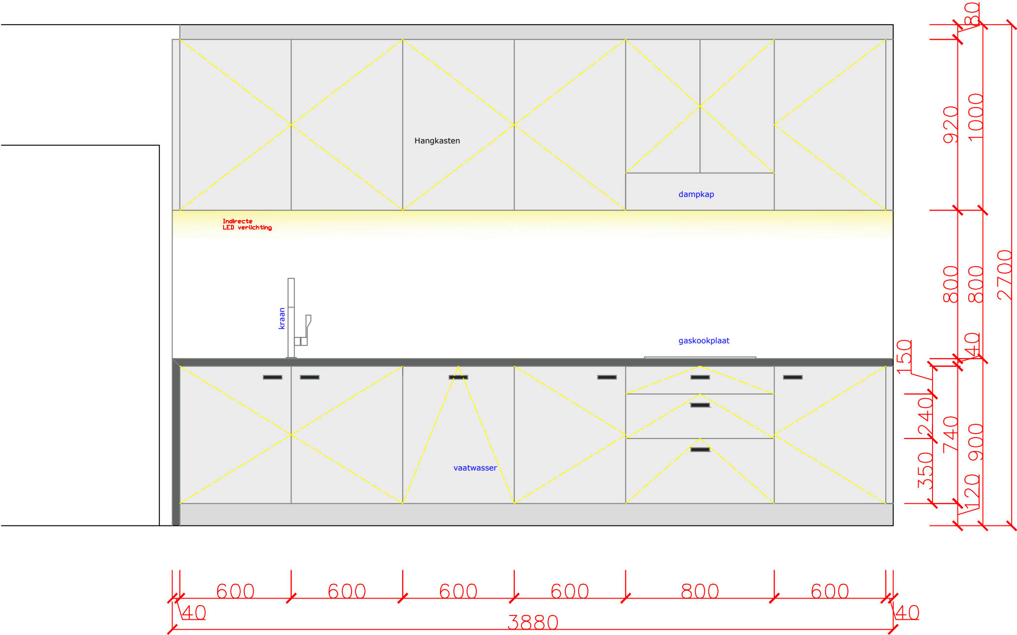
Kastindeling
