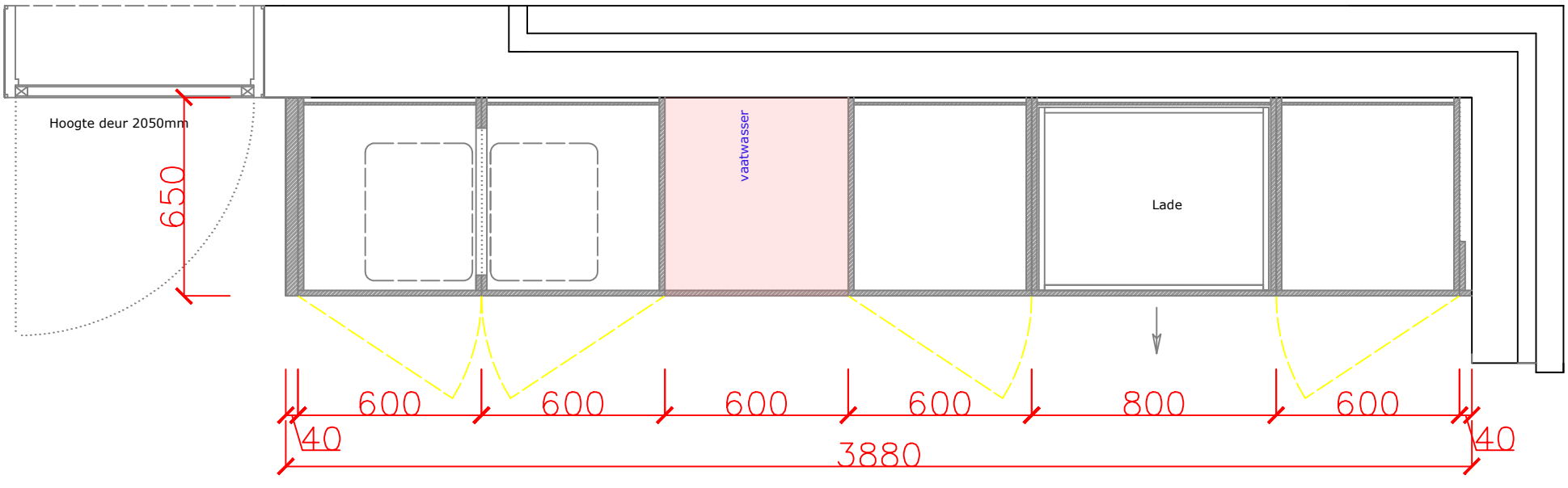
Grondplan onderkasten
