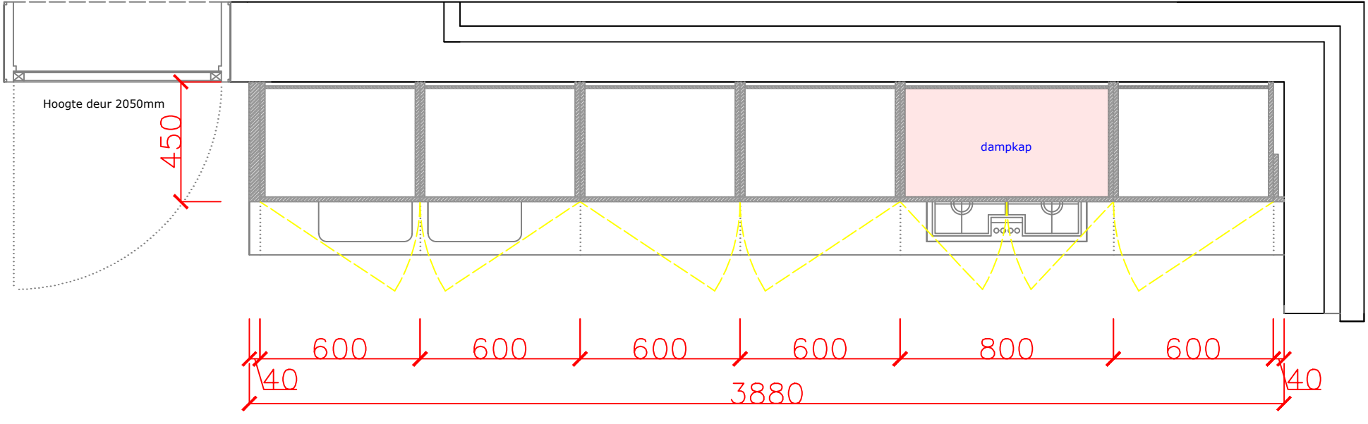
Grondplan hangkasten
