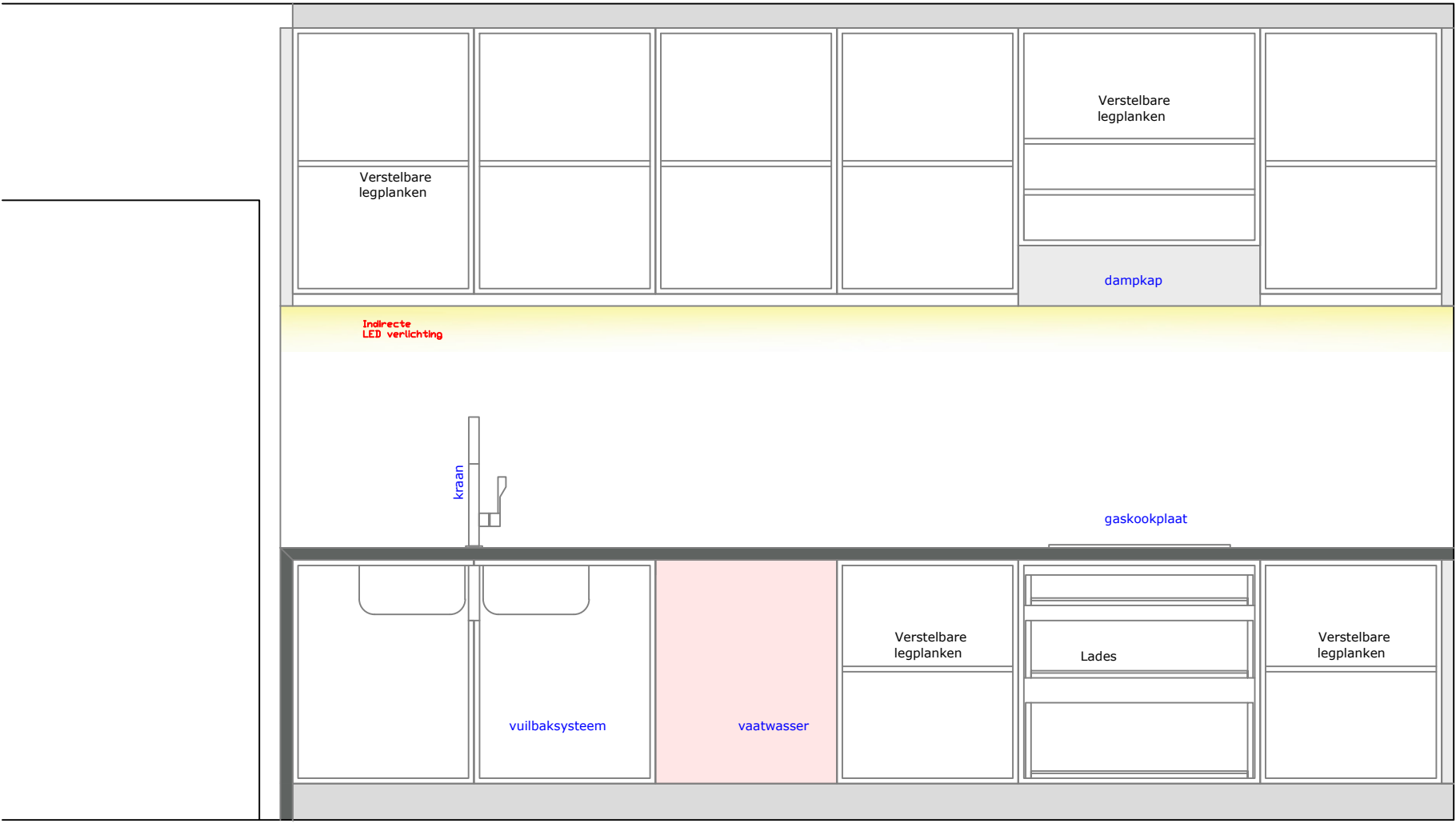
Kastindeling
